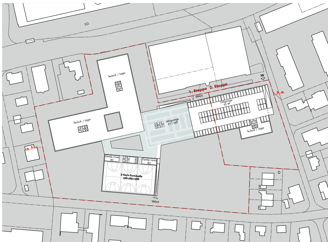
Grundriss Untergeschoss
